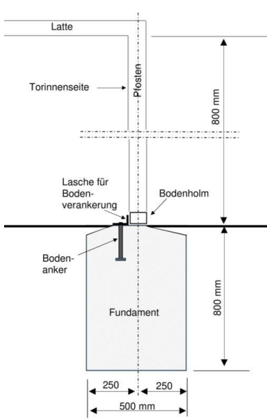
Beispiel 3 Fundament Schnitt B-B:
