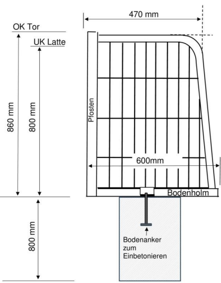
Beispiel Fundament Schnitt A-A:
