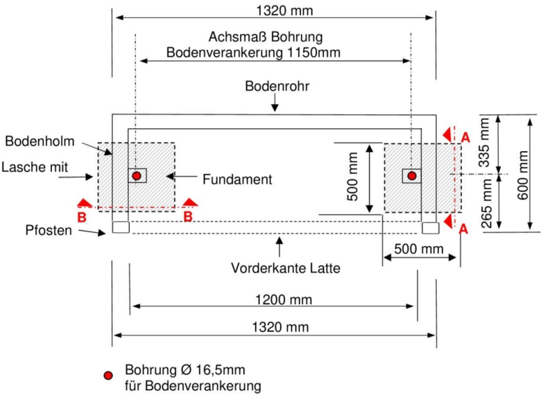
Beispiel Fundamentplan:
