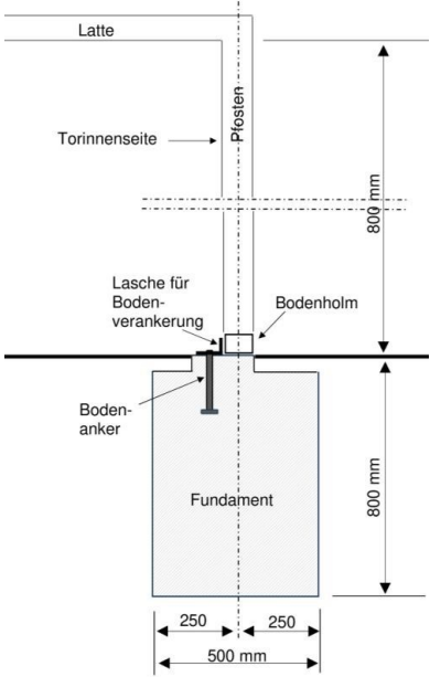
Beispiel 1 Fundament Schnitt B-B:
